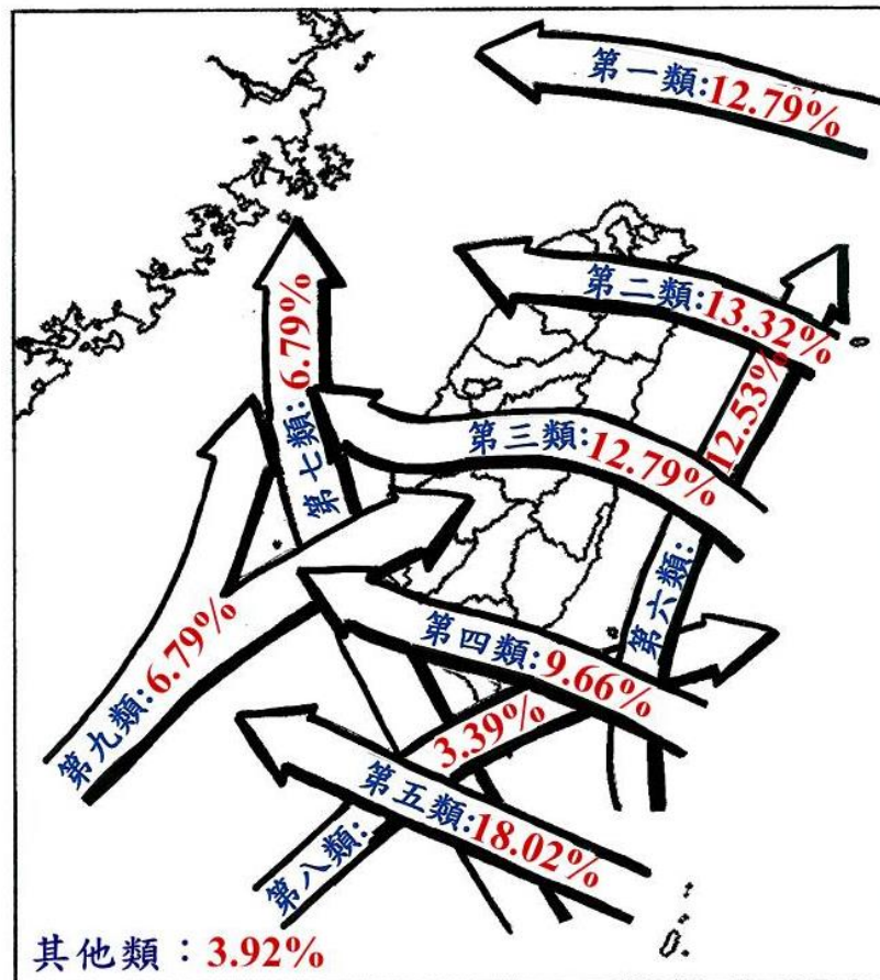
圖 2 影響臺灣地區颱風路徑分類圖
